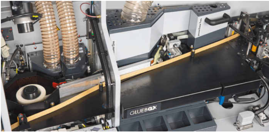
/ Startklar in nur 90 Sekunden: Bei der Kantenanleimmaschine Format4 Tempora F600 60.06L mit GlueBox verschmilzt ein dünner PUR-Klebestreifen Werkstück und Kantenmaterial nahezu unsichtbar miteinander.
